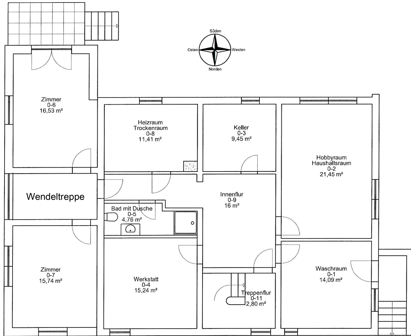
Kellergeschoss
