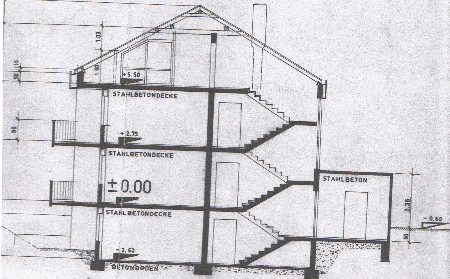
SCHNITT A-A'
